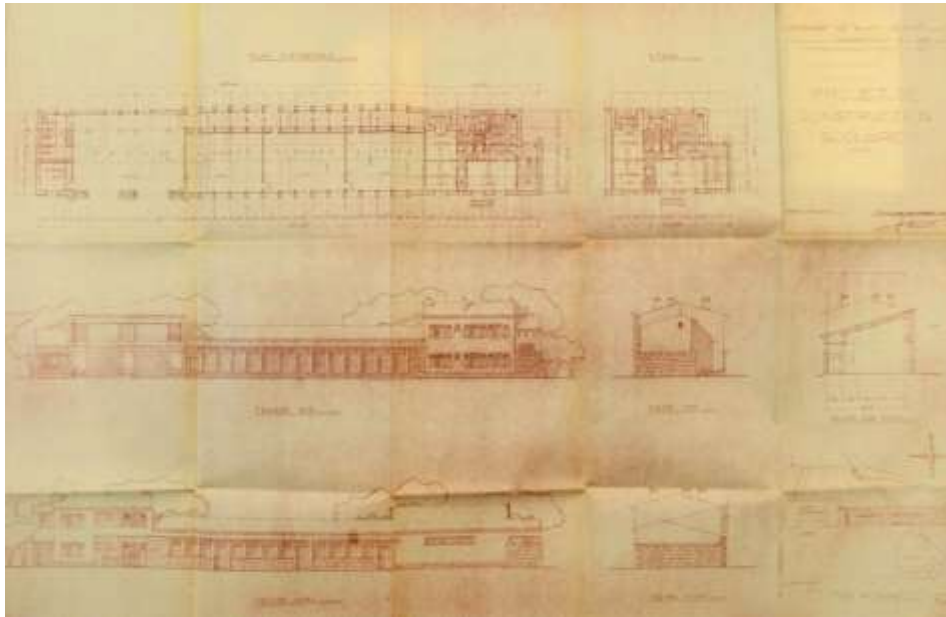
Illustration 20. Bernard Henri, projet d'agrandissement de l'école des garçons, plan d'ensemble, façades, coupes, 1955. Papier, dessin, 105 x 68,5 cm. Archives Départementales du Var, 2 Op 117/2.
