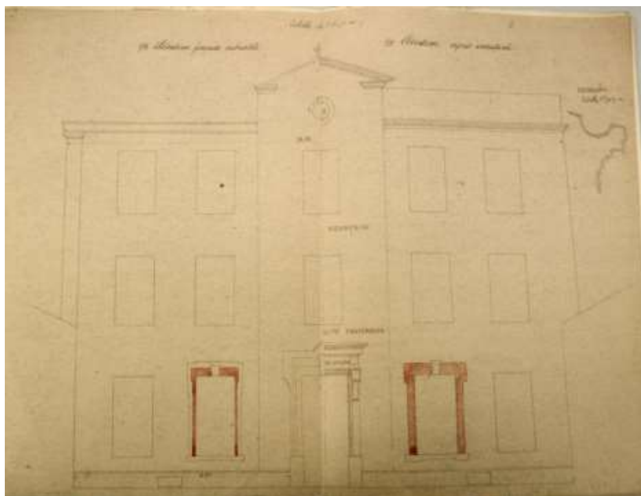
Illustration 19. Maneille, Aménagement de la Maison Planque en école de garçons, élévation façade actuelle, élévation façade après exécution, 1904.
